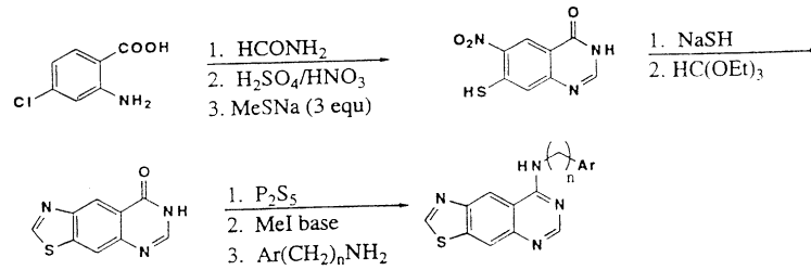
Schema 5. Sinteză grupe 6 preferate, fuziunea inelului [4,5-g].
