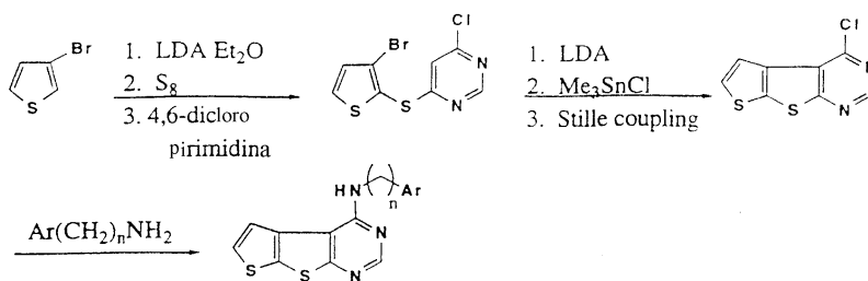
Schemă 19. Sinteza grupei preferate 41; fuziunea inelului [2',3':2,3] [5,4-d].
