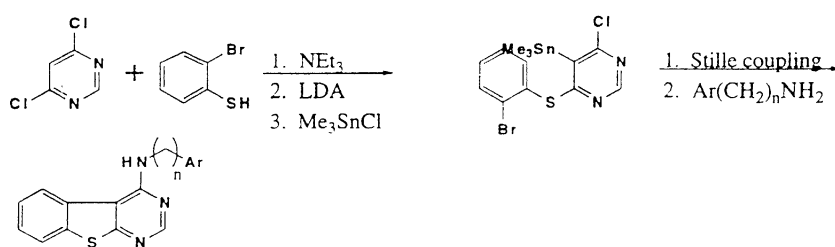
Schema 17. Sinteză grupei preferate 39; fuziunea inelului [2,3-d].
