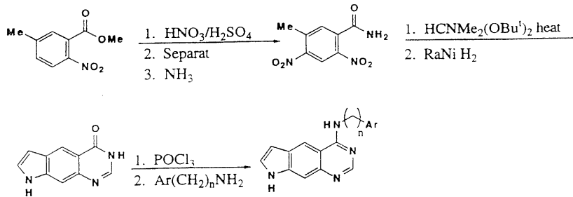
Schema 2. Sinteza grupei preferate4; fuziunea inelului [3,2-g].
