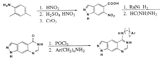
Schemă 8. Sinteză grupe 10 preferate; fuziunea inelului [4,3-g]
