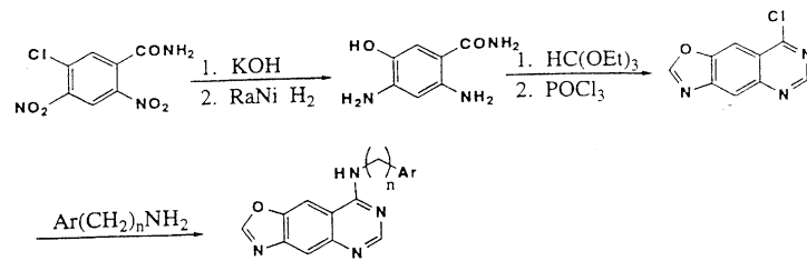
Schema 4. Sinteză grupe 5, fuziunea inelului [5,4-g].
