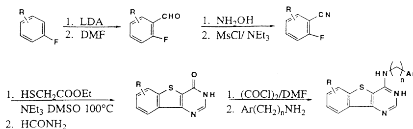
Schema 16. Sinteză grupei preferate 39; fuziunea inelului [3,2-d]
