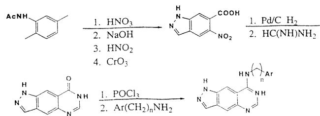
Schemă 9. Sinteză grupe 10 preferate; fuziunea inelului [3,4-g]
