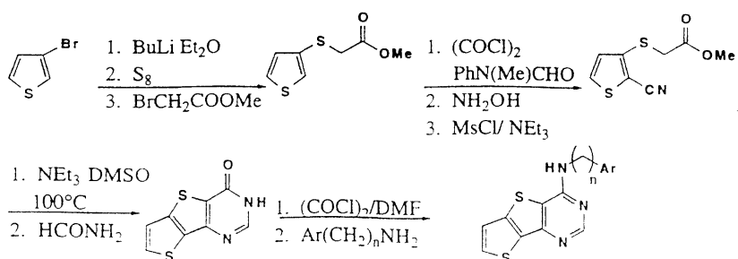
Schema 18. Sinteză grupei preferate 41; fuziunea inelului [3',2':2,3] [4,5-d].
