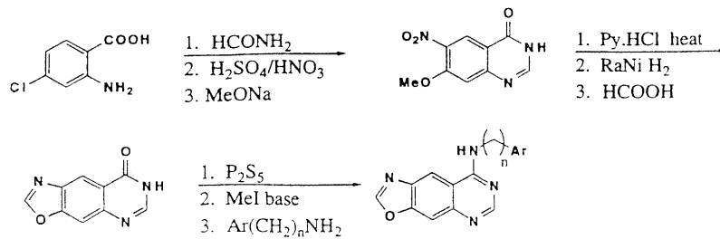
Schema 3. Sinteza grupei preferate5; fuziunea inelului [4,5-g].
