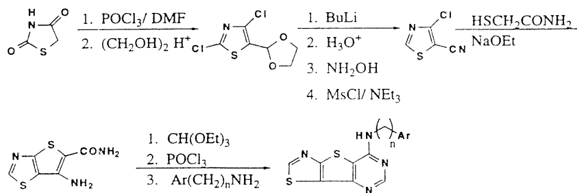
Schemă 20. Sinteza grupei preferate 44; fuziunea inelului [4',5':2,3] [4,5-d].
