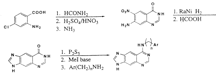
Schemă 7. Sinteză grupe 7 preferate
