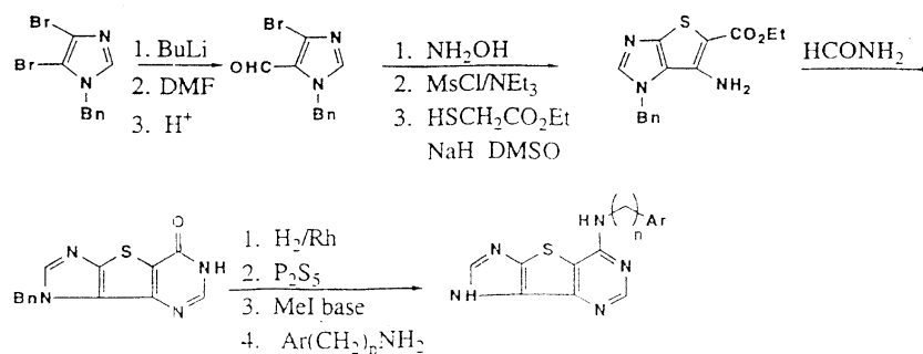
Schemă 21. Sinteza grupei preferate 45; fuziunea inelului [4',5':2,3] [4,5-d].
