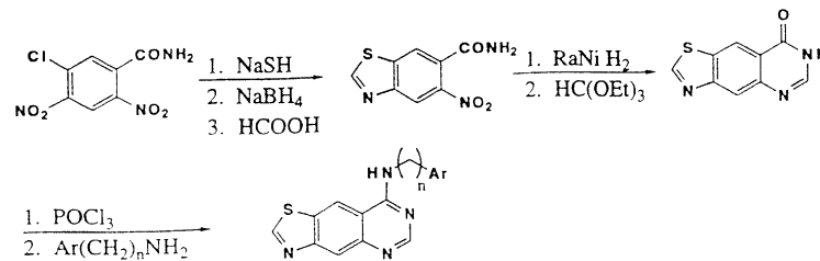
Schema 6. Sinteză grupe 6 preferate, fuziunea inelului [5,4-g].
