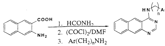
Schema 1. Sinteza grupei preferate1.
