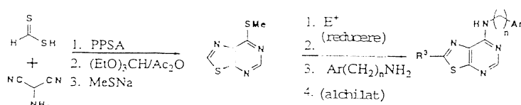
Schema 23. Sinteza grupei preferate 44; fuziunea inelului [5,4-d].
