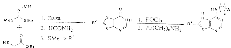
Schema 24. Sinteza grupei preferate 44; fuziunea inelului [4,5-d].
