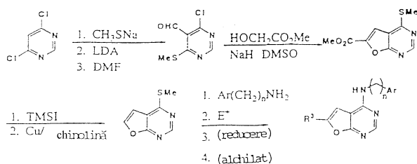
Schema 20. Sinteză grupe preferate 42; fuziunea inelului [2,3-d]
