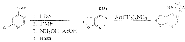
Schema 28. Sinteză grupei preferate 47; fuziunea inelului [5,4-d].
