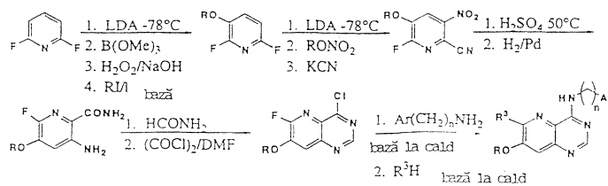
Schema 3. Sinteză grupelor preferate 6 și 8-10; R 4 = RO
