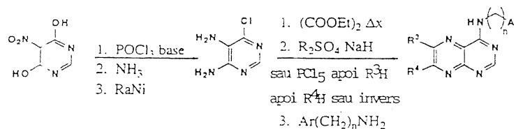
Sch. nr. 16. Sinteza grupelor preferate 37-40.
