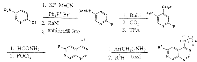
Schema 8. Sinteza grupelor preferate 17-21.
