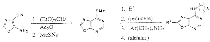
Schema 25. Sinteză grupei preferate 45; fuziunea inelului [5,4-d].
