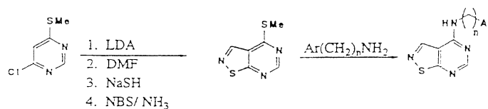
Schema 30. Sinteză grupei preferate 48; fuziunea inelului [5,4-d].
