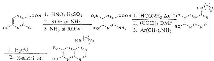
Schemă 13. Sinteză grupelor preferate 29 și 30; R 4 = CR
