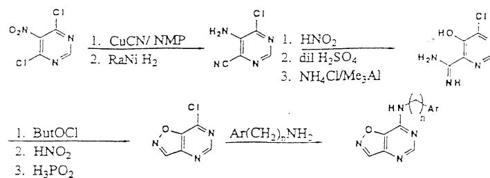
Schema 29. Sinteză grupei preferate 47; fuziunea inelului [4,5-d].
