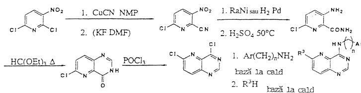
Schema 1. Sinteză grupelor preferate 1-5; R 4 = H
