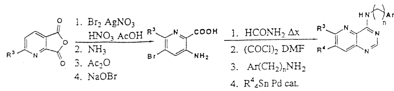
Schema 4. Sinteza grupei preferate 7.
