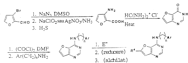
Schema 19. Sinteză grupe preferate 42; fuziunea inelului [2,3-d]
