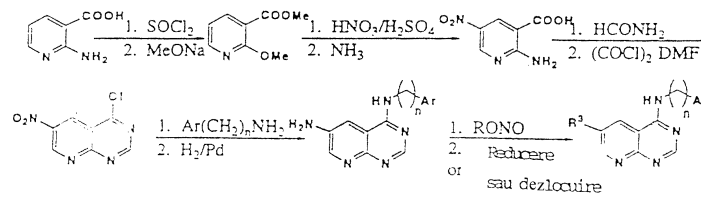
Schema 9. Sinteza grupelor preferate 22-26; R 4 = H.
