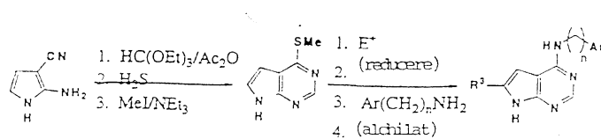
Schema 21. Sinteza grupei preferate 43; fuziunea inelului [2,3-d]
