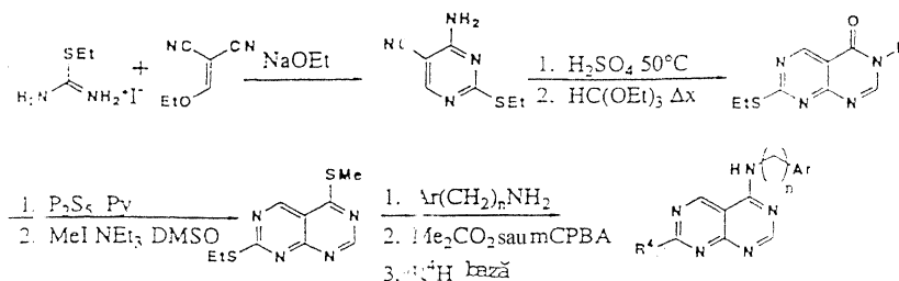
Sch. nr. 15. Sinteza grupelor preferate 33-36.
