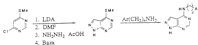
Schema 32. Sinteză grupei preferate 49; fuziunea inelului [3,4-d].
