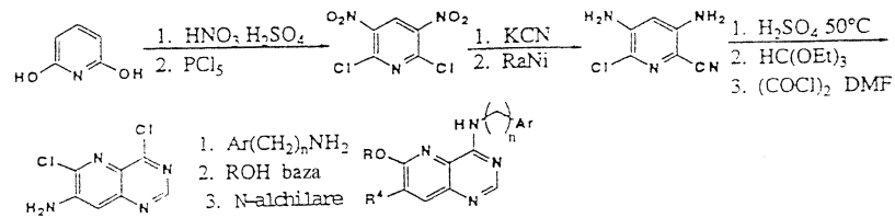
Schema 5. Sinteza grupelor preferate 8 si 9; R^3 = OR .
