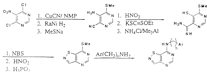
Schema 31. Sinteză grupei preferate 48; fuziunea inelului [4,5-d]
