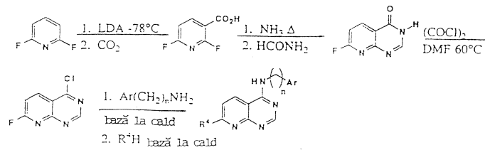
Schema 10. Sinteza grupelor preferate 22-26; R 3 = H.
