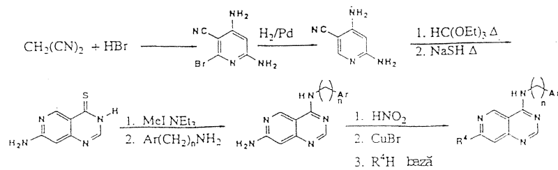
Schema 7. Sinteza grupelor preferate 12-16.
