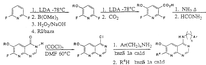
Schemă 11. Sinteză grupelor preferate 27 și 29-31; R 3 = RO
