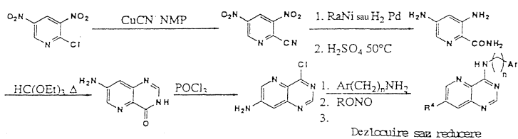
Schema 2. Sinteză grupelor preferate 1-5; R 3 = H
