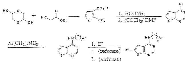
Schema 18. Sinteză grupe preferate 41; fuziunea inelului [2,3-d]
