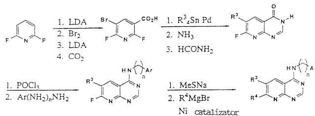
Schemă 12. Sinteză grupe preferate 28.
