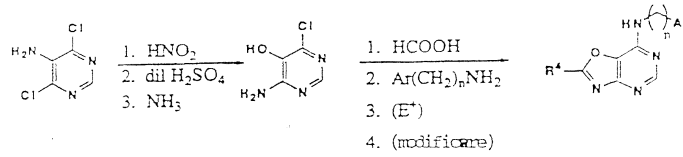
Schema 26. Sinteză grupei preferate 45; fuziunea inelului [4,5-d].
