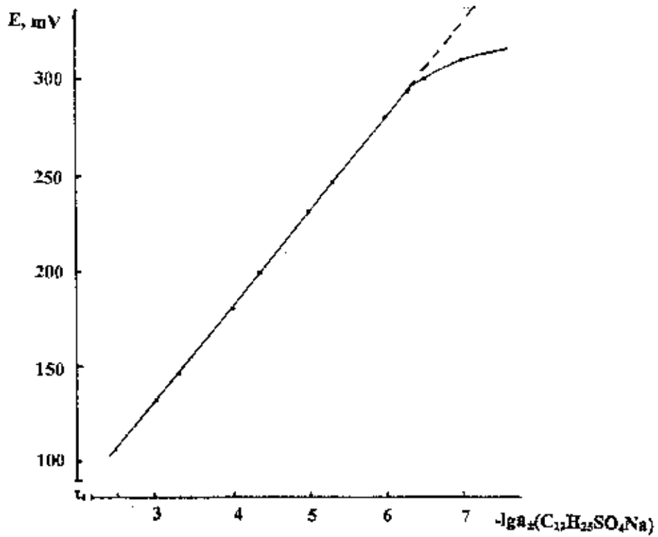
Dependența potențialului E al elementului galvanic de valoarea negativă a logaritmului activității dodecilsulfatului de sodiu
