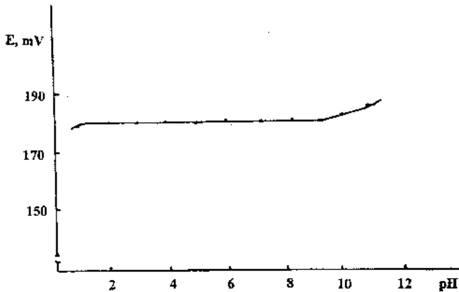
Influența pH-ului asupra potențialului electrodului introdus în soluția de dodecilsulfat de sodiu cu concentrația 10^{-4} mol/L
