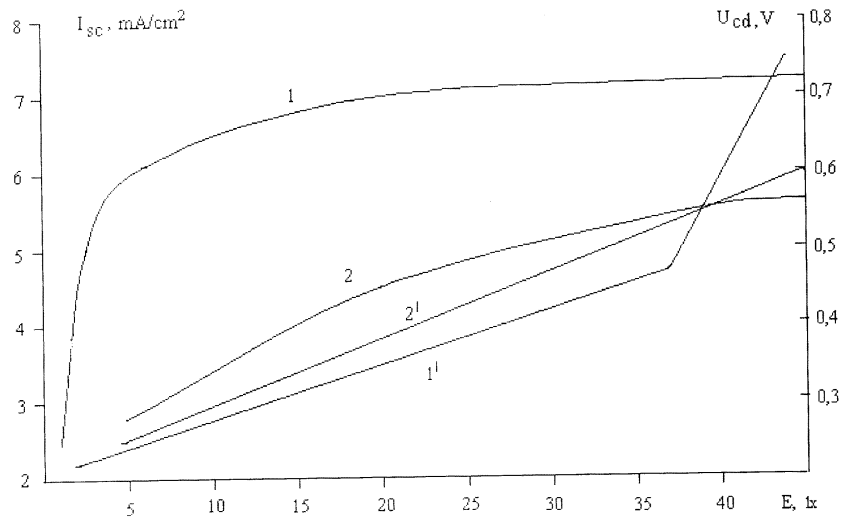
Dependenta I_{sc} și U_{cd} de intensitatea iluminării
