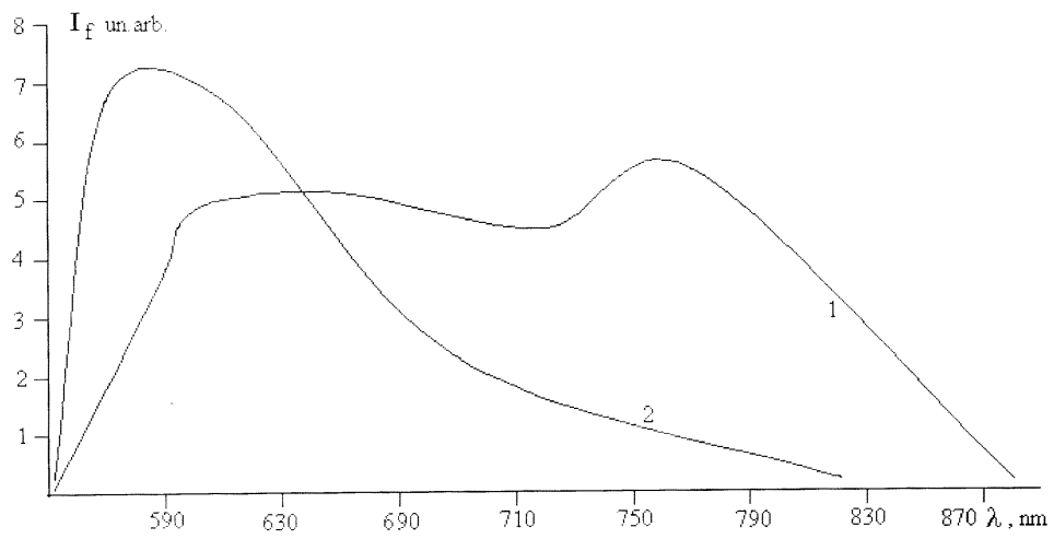
Distribuția spectrală a heterostructurilor ZnTe-CdSe ; 1- HS de tip I 2- HS de tip II
