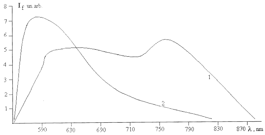
Distribuția spectrală a heterostructurii lor ZnTe-CdSe ; 1- HS de tip I 2- HS de tip II
