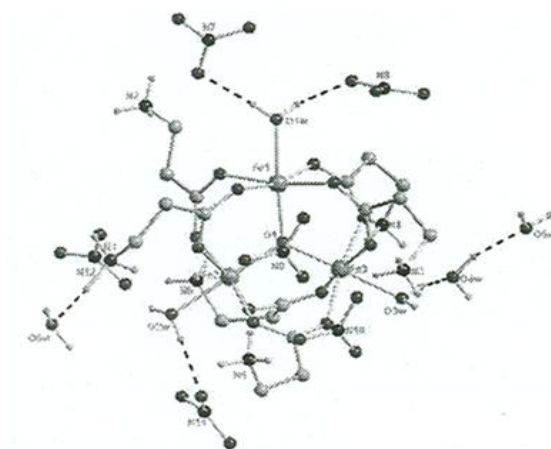
Structura moleculară a \beta -alaninului oxotrinuclear de fier(III)
