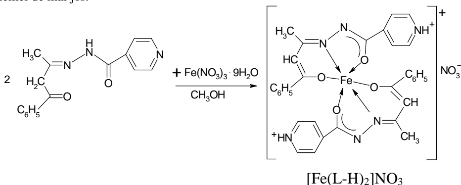
Schema 1. Obținerea compusului [\text{Fe}(\text{L}-\text{H})_2]\text{NO}_3
