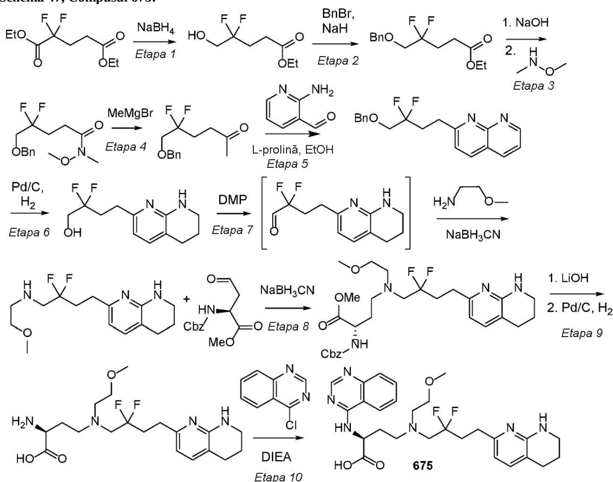
Schema 47, Compusul 675:
